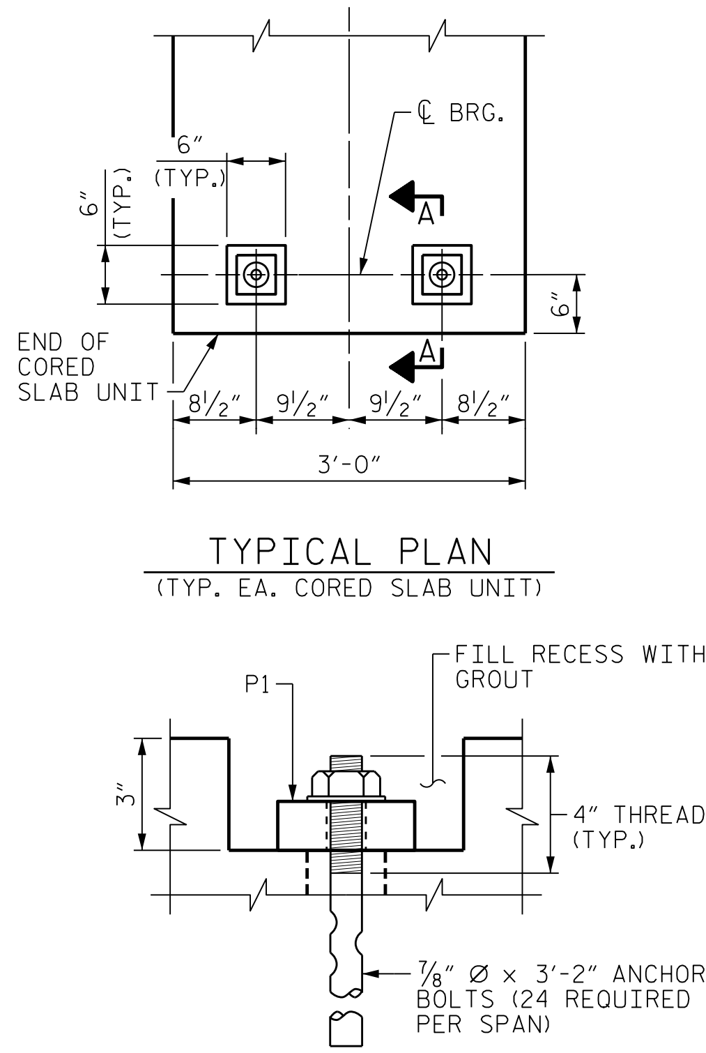
SECTION A-A
